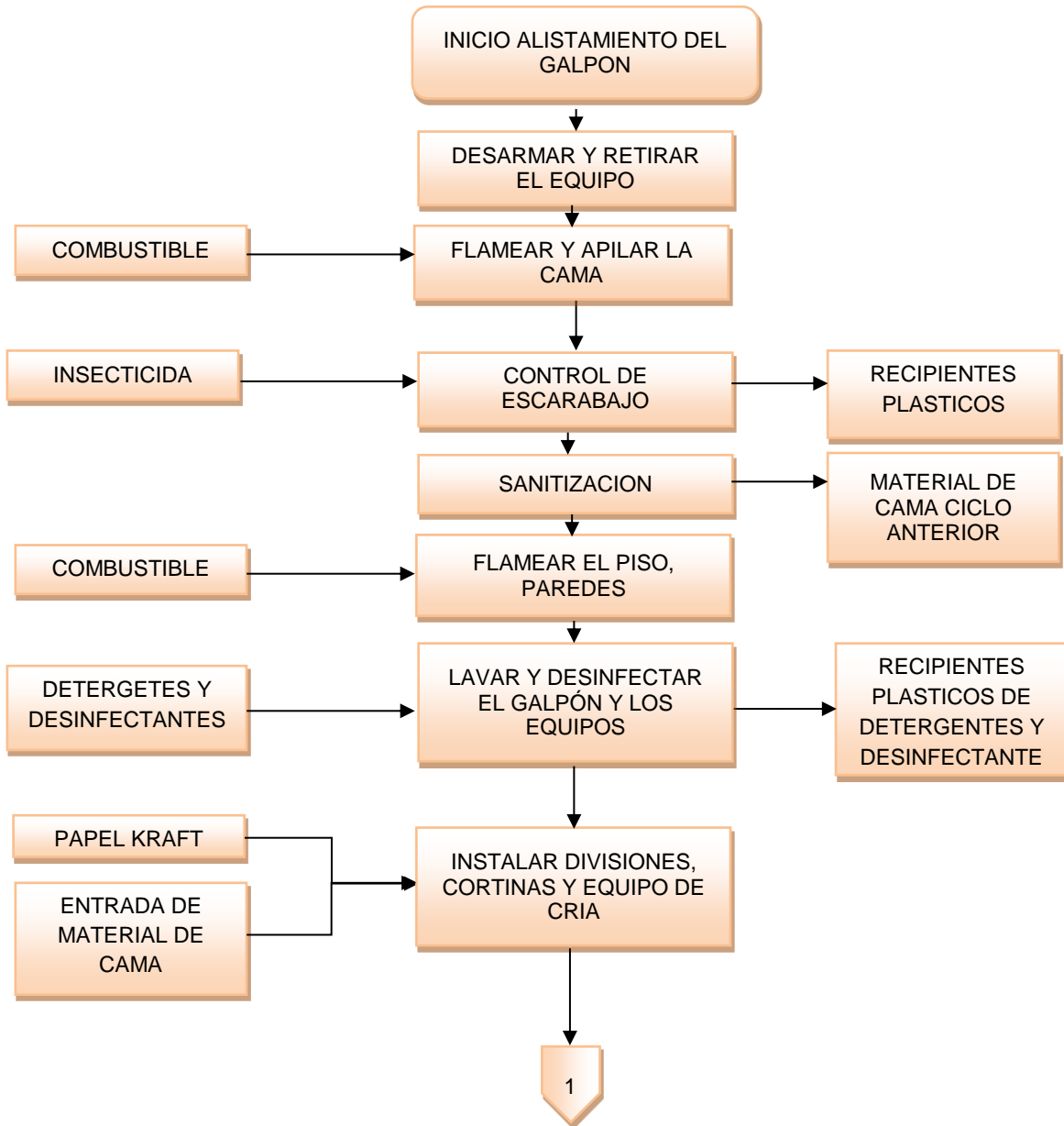
Figura 1. Diagrama de Flujo Granja San Roque
